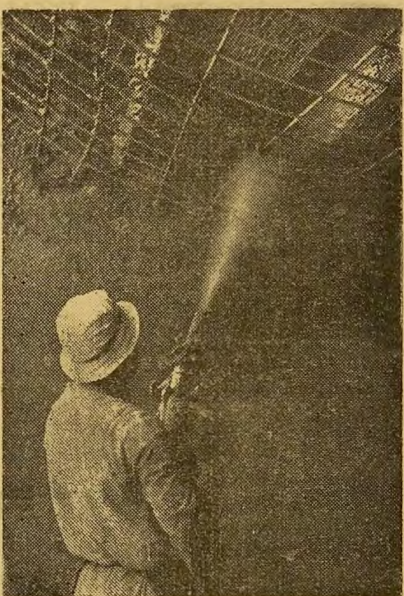
La projection du mortier à «Gunit»
